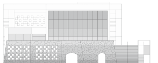
決定した護佐丸歴史資料図書館の建物外観(正面図)
